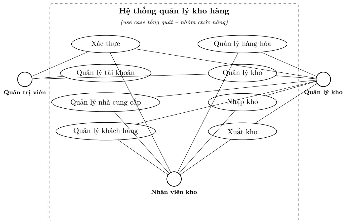
Figure 1: Sơ đồ use case tổng quát (nhóm chức năng – chưa phải UC chi tiết)
